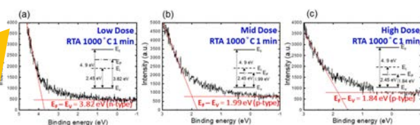
以UPS量測費米能階，並證實可以用磷離子植入達到p-type \text{Ga}_2\text{O}_3
